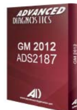
Logiciel ADS2187
